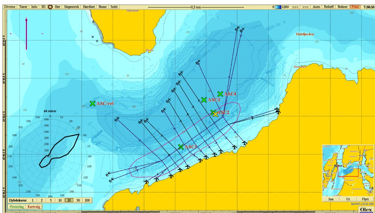
Figur 2: Kartet viser anleggsplassering, modellert AZE og ASC-stasjoner ved Skonseng. Lilla pil viser orientering av kart, strømrose viser vanntransport ( m^3/m^2/døgn ) for hver 15° sektor på 64 meters dyp (spredningsdyp), og gult kryss markerer posisjon for strømmålingene i 2020-2021 ( 65^{\circ}48.610'N , 12^{\circ}37.720'Ø ; Nergaard, 2021). Målestokk vises øverst i bildet. Kilde: Olex. Kartdatum WGS84.
