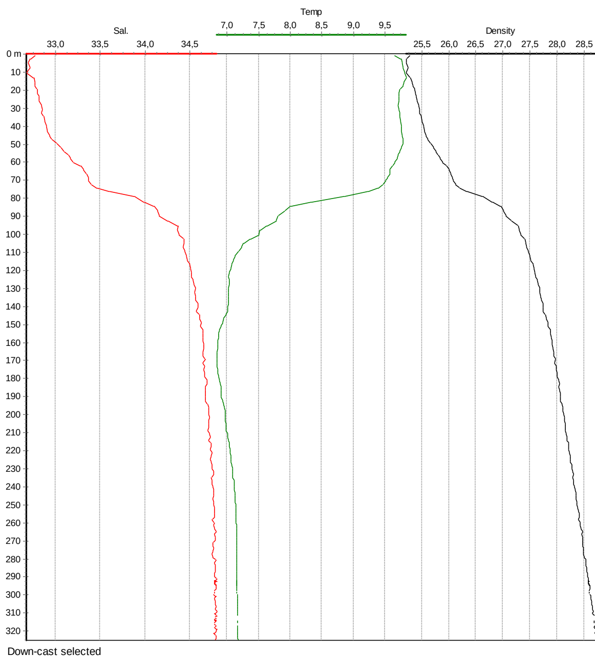
Figur 4: Sjøtemperatur (°C; grønn), salinitet (rød) og tetthet ( -1000 \text{ kg/m}^3 ; sort) fra overflaten og ned til bunnen (down-cast) på 325 meters dyp ved stasjon C2 den 23.10.2019.
